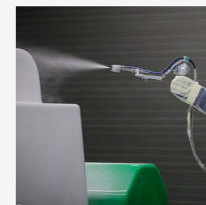
2. Application du gelcoat, qui donnera la couleur du bassin
